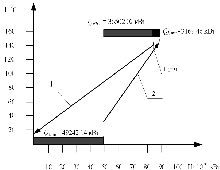
Рис. 4. Составные кривые для интегрированного процесса при \Delta T_{\min} = 6^{\circ}\text{C} : 1 – горячая составляющая кривая, 2 – холодная составляющая кривая; Q_{H\min} – горячие утилиты; Q_{C\min} – холодные утилиты; Q_{REC} – мощность рекуперации
